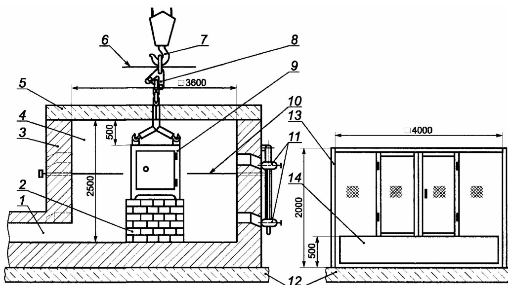
Установка для испытаний сейфов на огнестойкость
